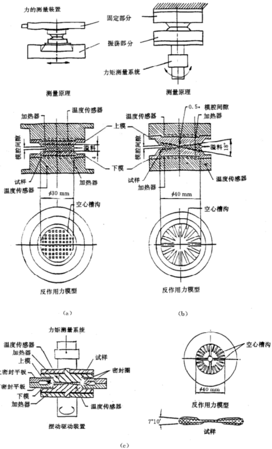
图 2 硫化仪的类型
